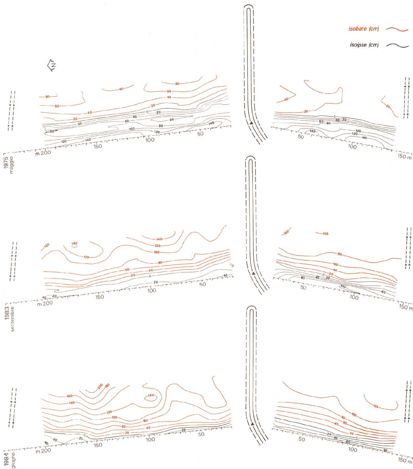
Tavola 10 – Rilievi altimetrici e batimetrici a ridosso del pennello antistante alla sezione 3cIV, relativi al maggio 1975, al settembre 1983 e al giugno 1984.
